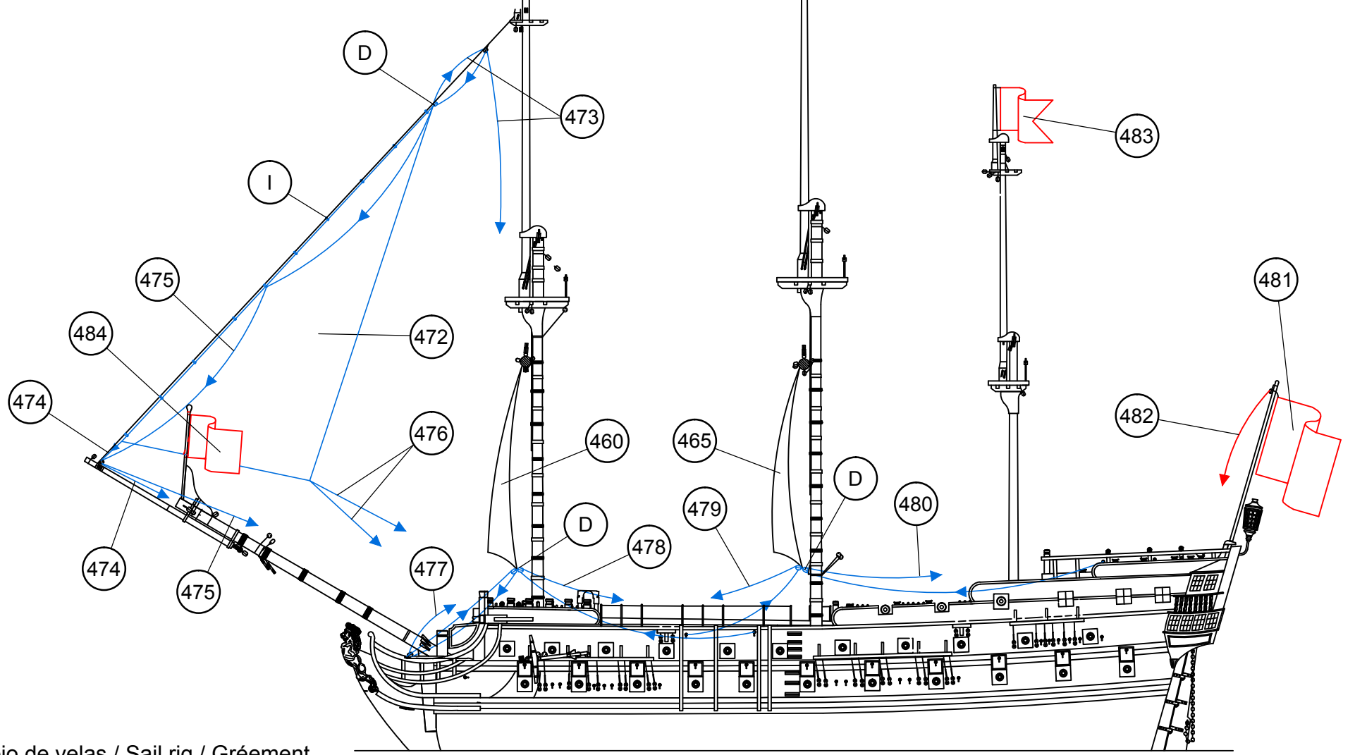
Aparejo de velas / Sail rig / Gréement Segel takelage / Sartieme da vela
